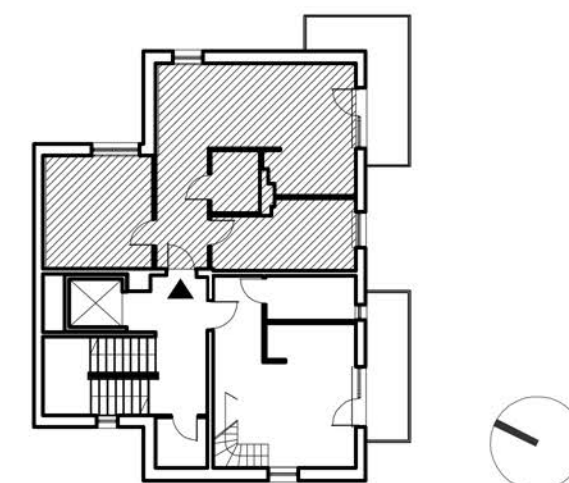
RZUT PIĘTRA I BUD. 'A'
