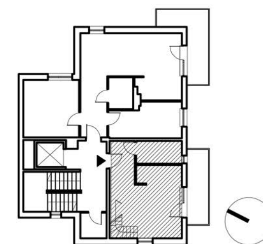
RZUT PIĘTRA I BUD. 'A'
