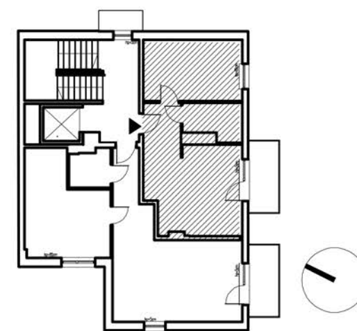
RZUT PIĘTRO I BUD. 'B'
