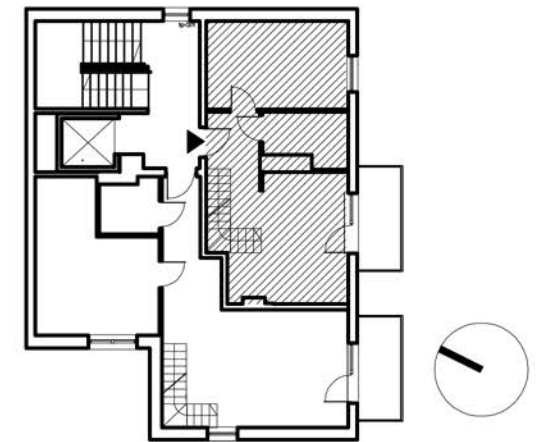
RZUT PIĘTRA II BUD. 'B'
